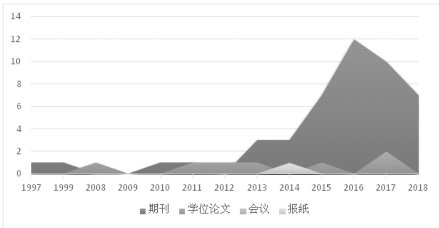
图1 文献数量情况统计图
