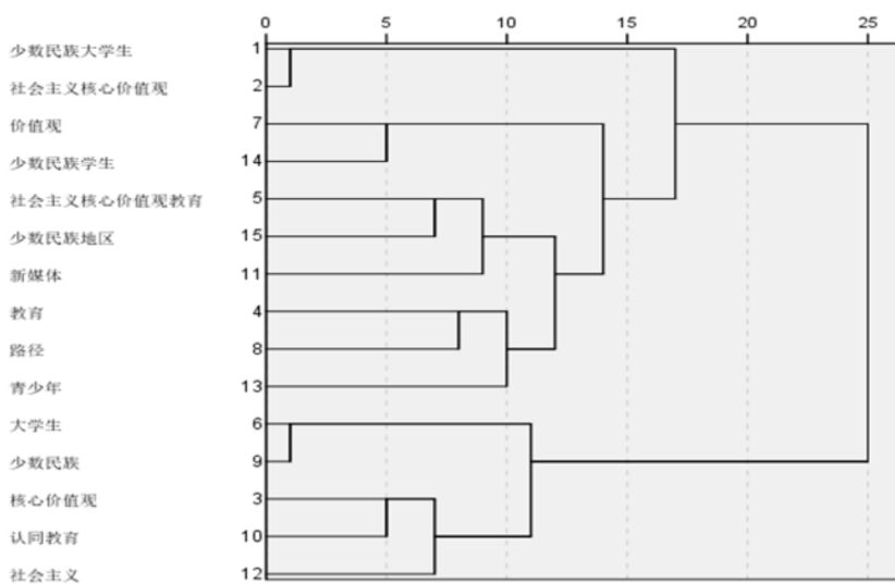
图 2 高频关键词聚类图
