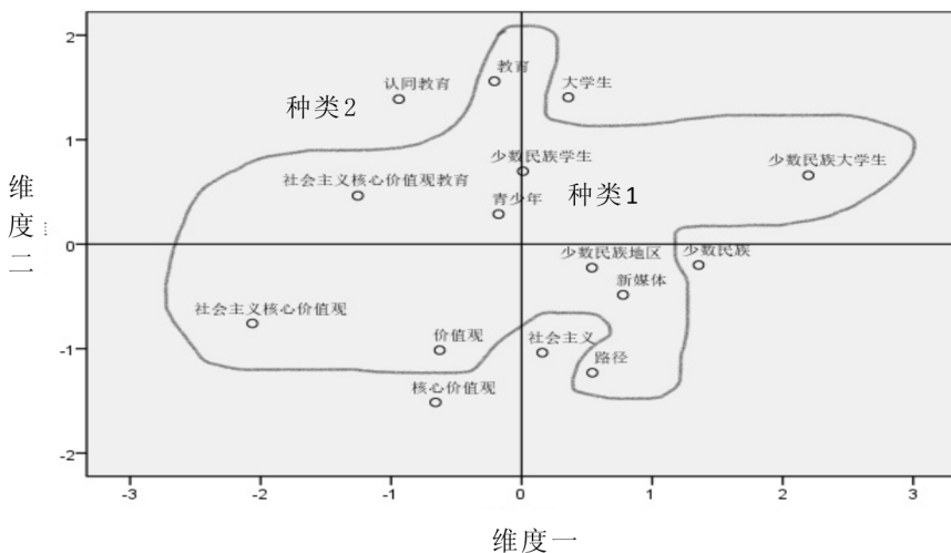
图3 研究热点可视化图谱(高频关键词)
